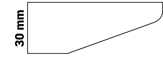
B20-R Canto con bisel a 20° y 1/2 caña de 10 mm
