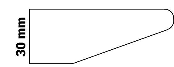
B20-M Canto con bisel a 20° y 1/4 de caña de 10 mm
